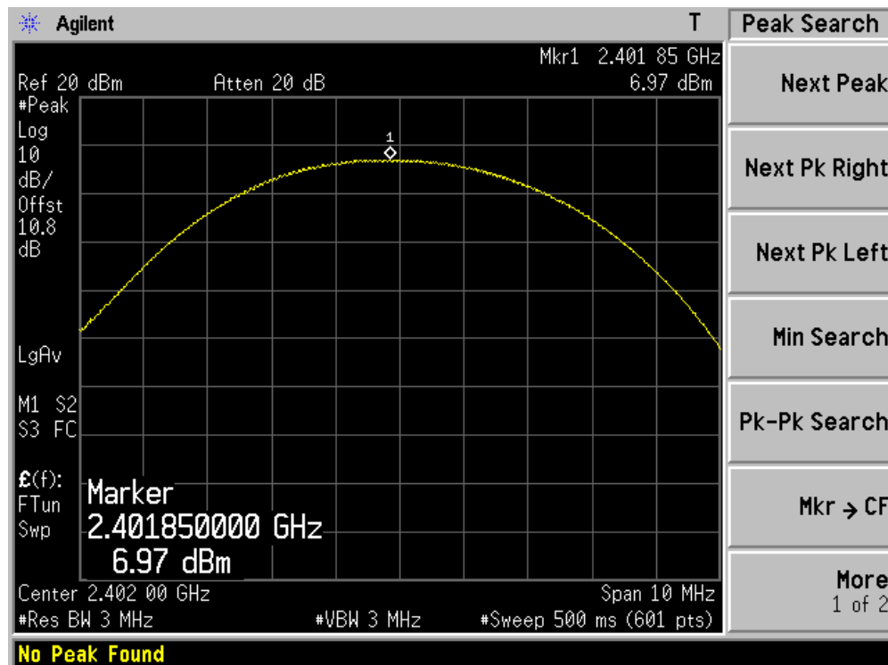
2DH5 2402MHz
