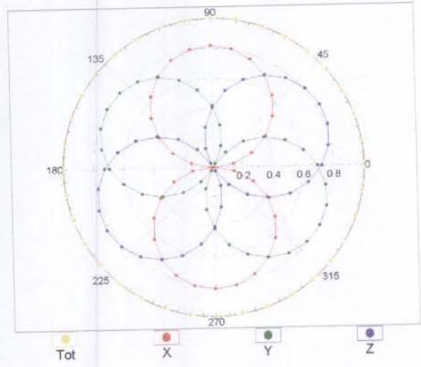
f=1800 MHz,R22
