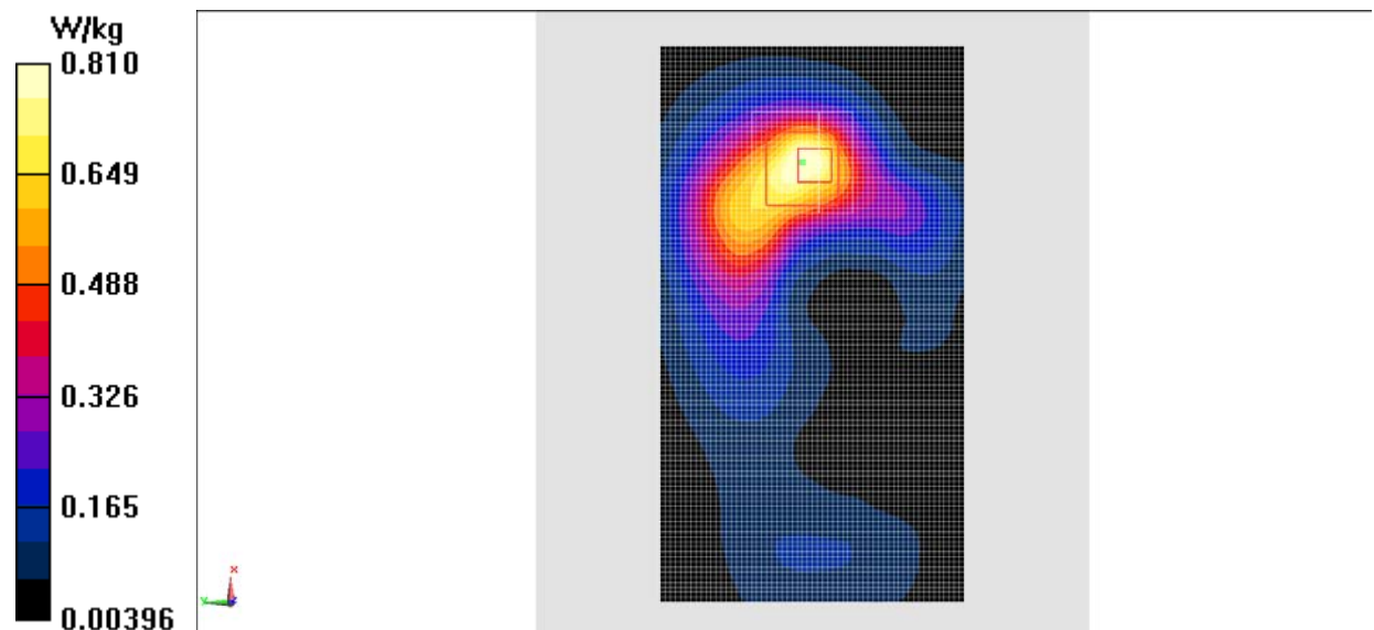
Fig.10 LTE Band7
