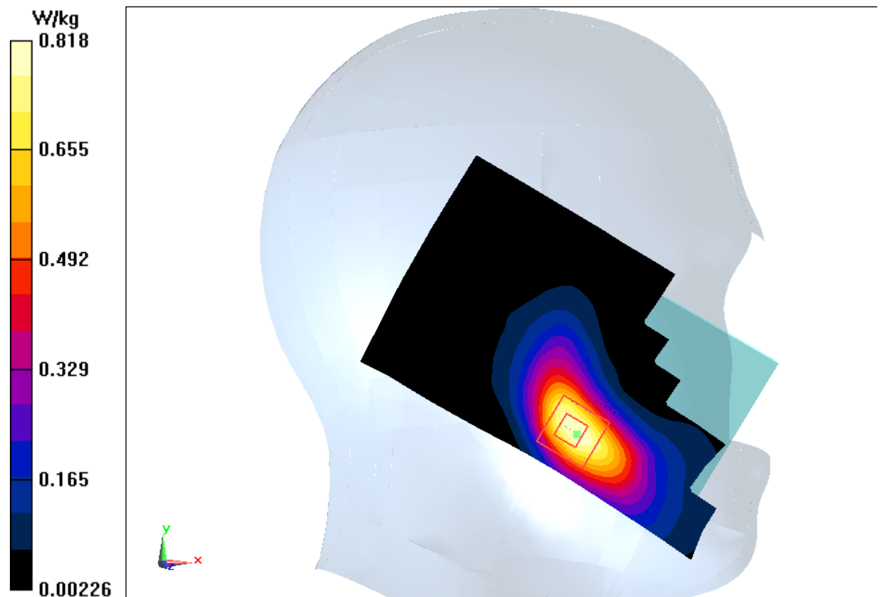
Fig.9 LTE Band7
