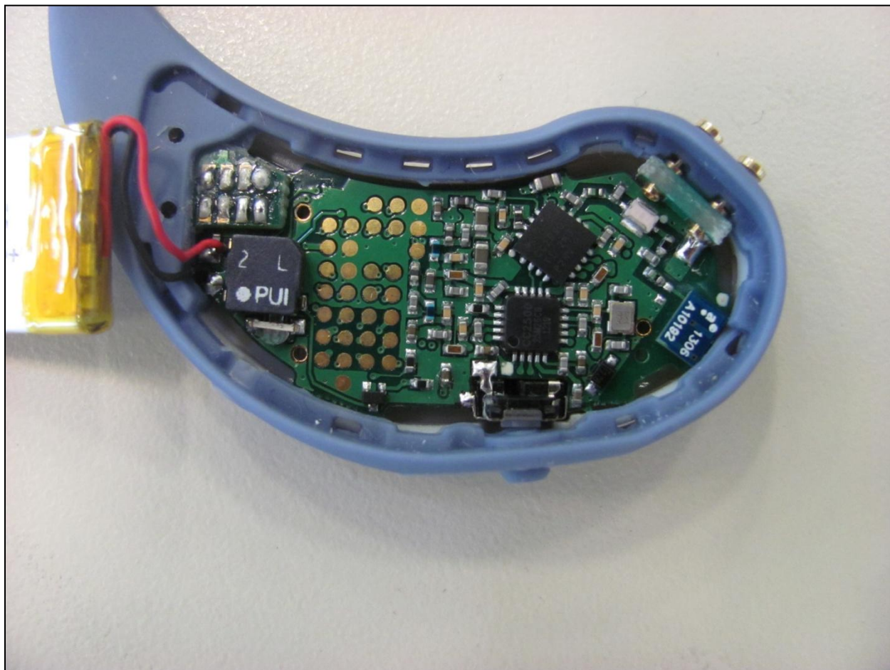
EUT – Photo 3
