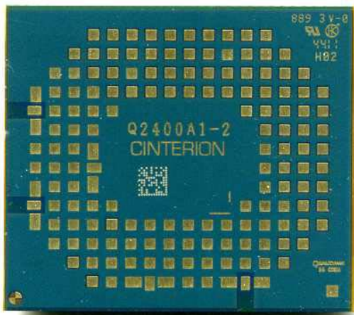
PXS8 Bottom Side
