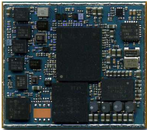
PXS8 Top side
