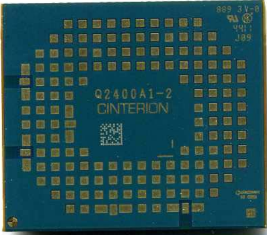
PVS8 Bottom Side
