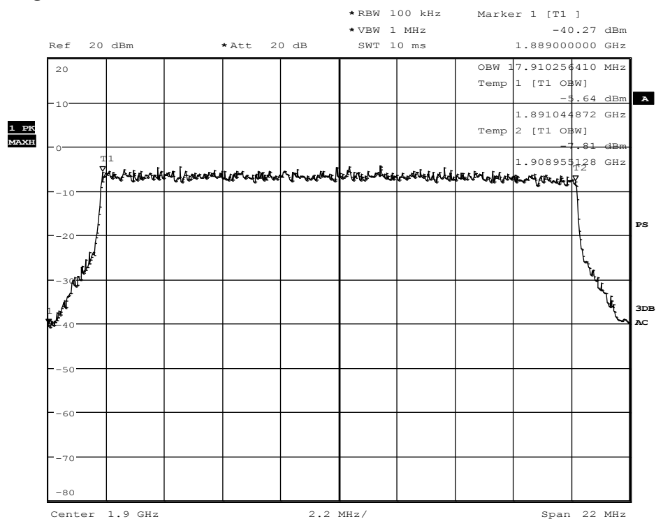
Diagram 35.216_OBW 20MHz Ch_18900
