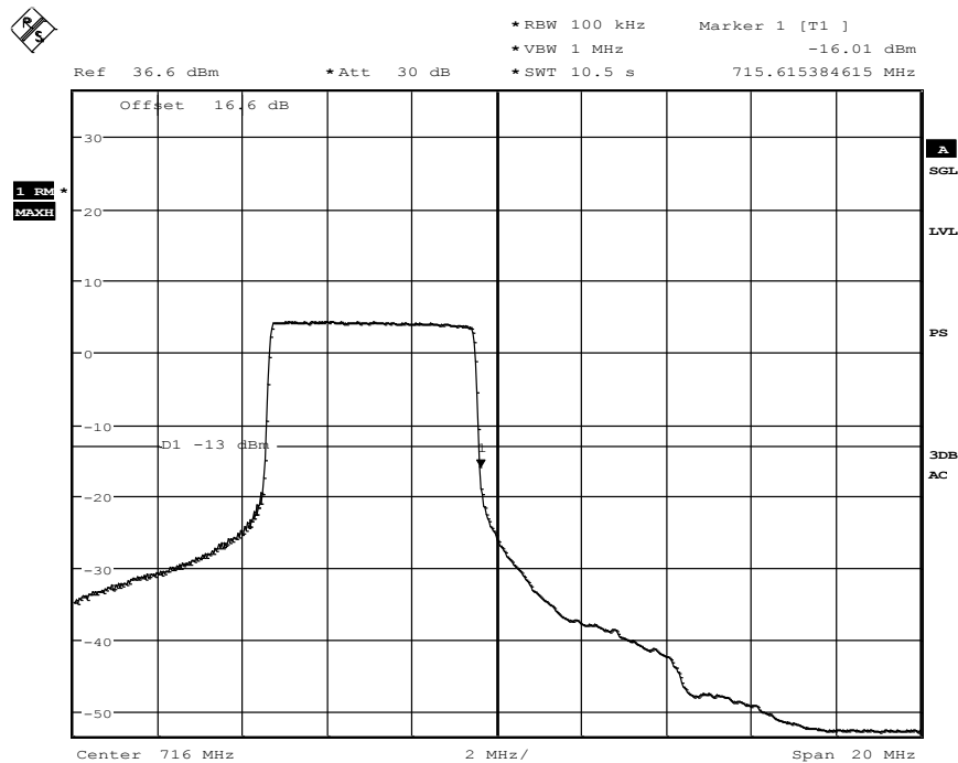
Diagram Ch 23130_QPSK_10MHZ
