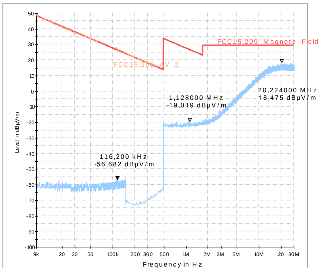
FCC15.209_magn hor+vert
