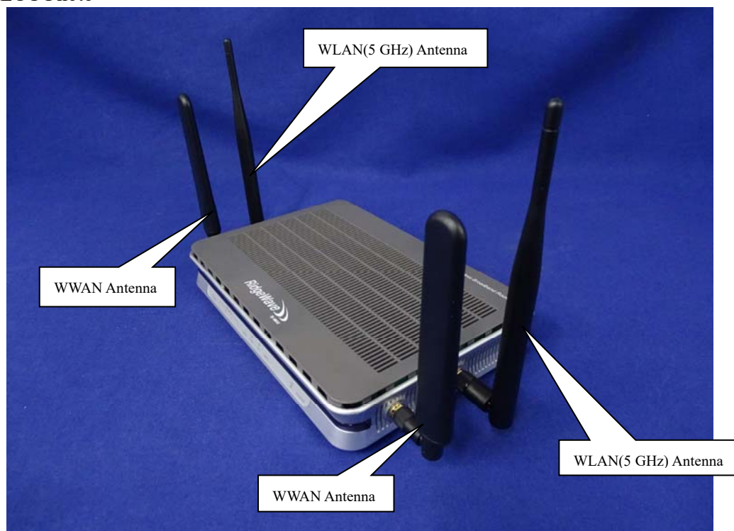
(9) EUT Photo
