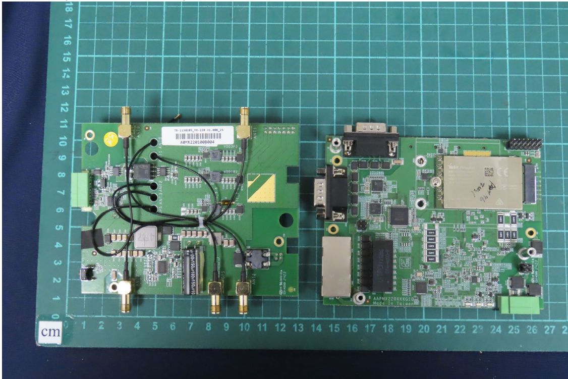
(5) EUT Photo (MX-220-UT-5G-A)
