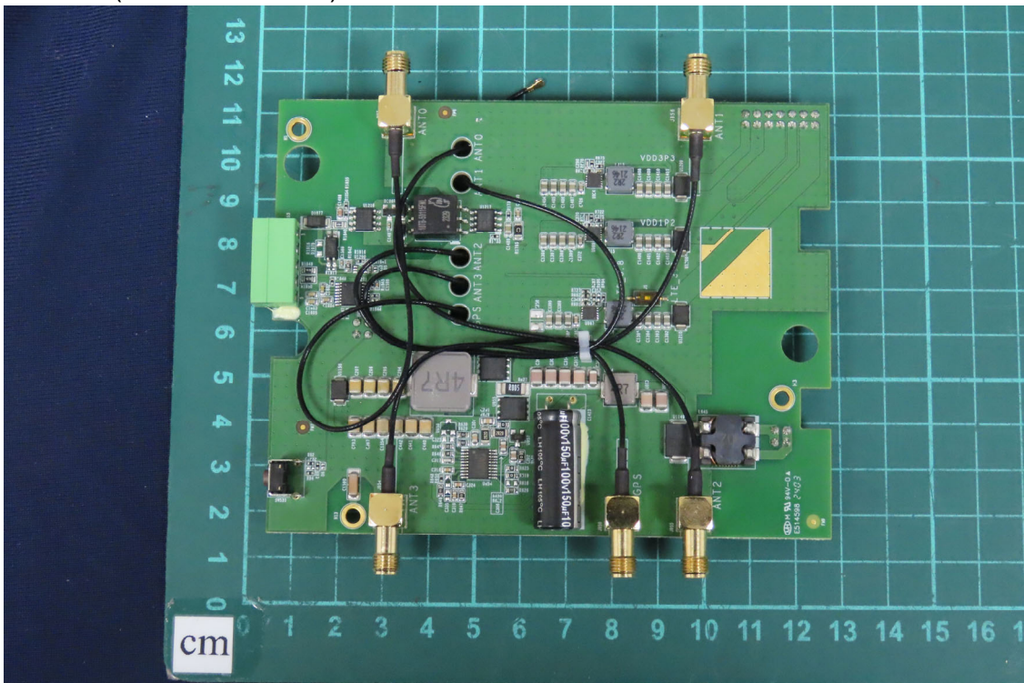
(6) EUT Photo (MX-220-UT-5G-A)
