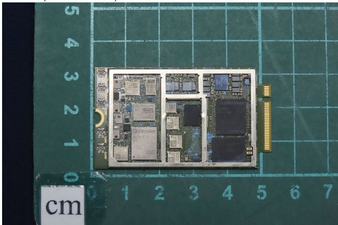
(12) EUT Photo (MX-220-UT-5G-A)
