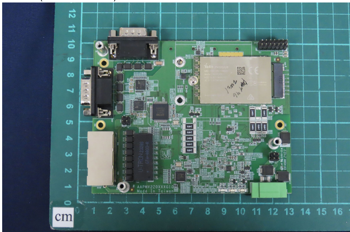
(8) EUT Photo (MX-220-UT-5G-A)
