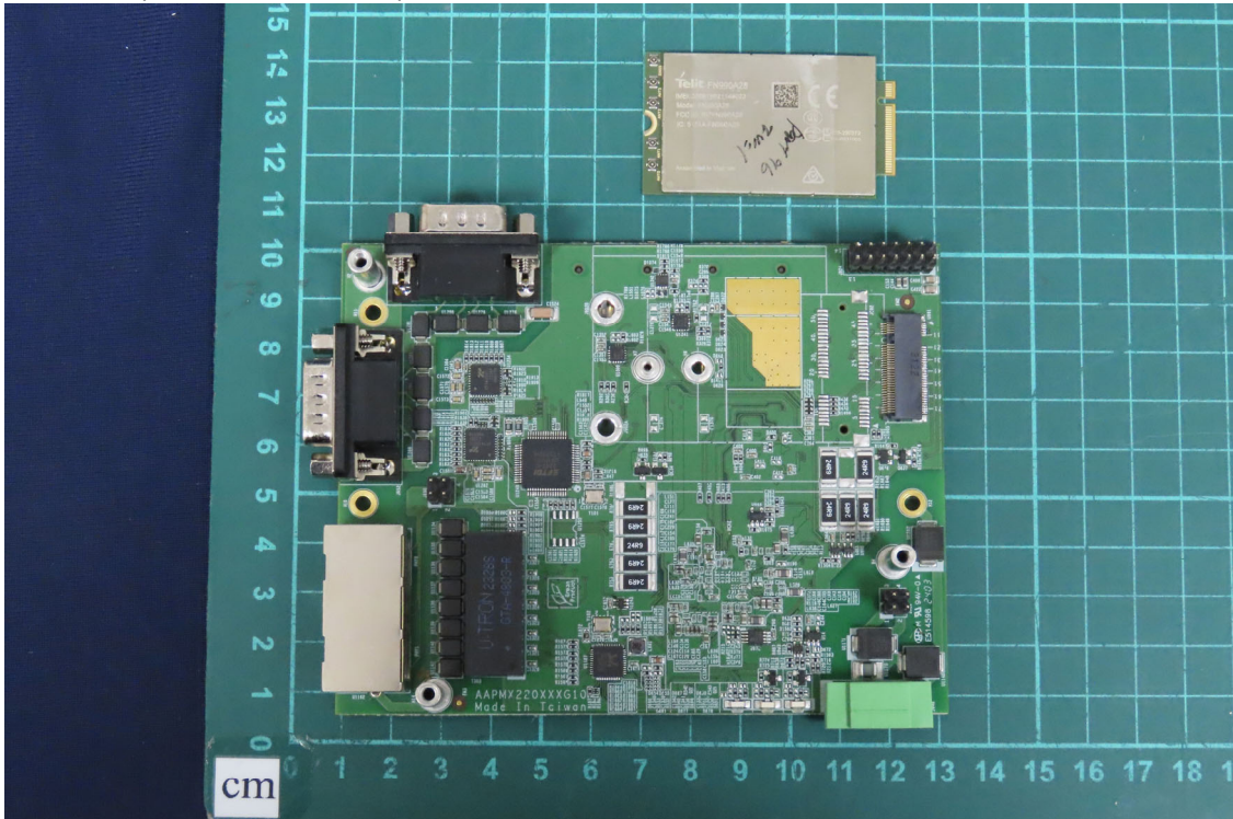
(9) EUT Photo (MX-220-UT-5G-A)
