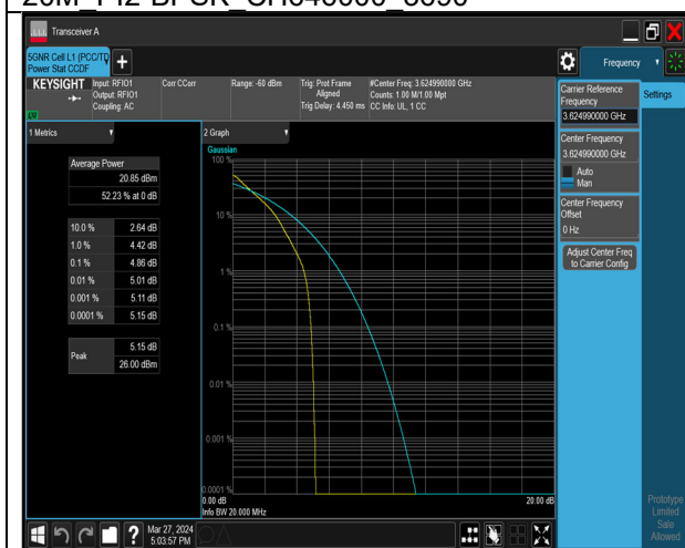
20M QPSK CH641666 3625
