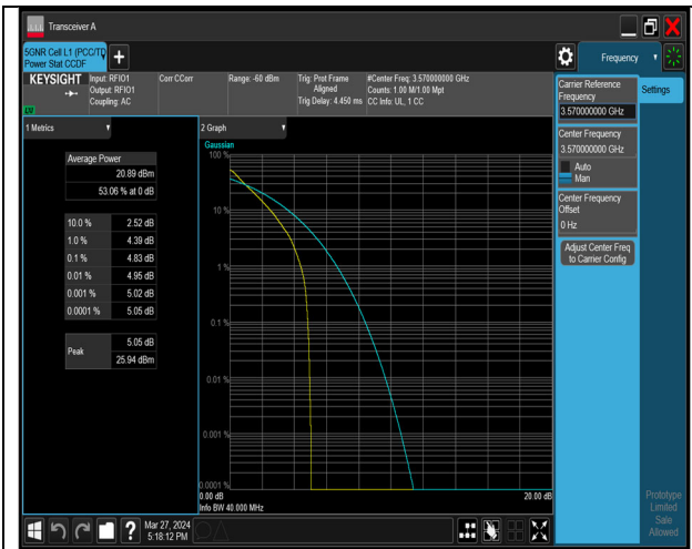
40M QPSK CH638000 3570
