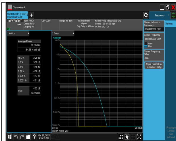
20M PI2-BPSK CH637334 3560
