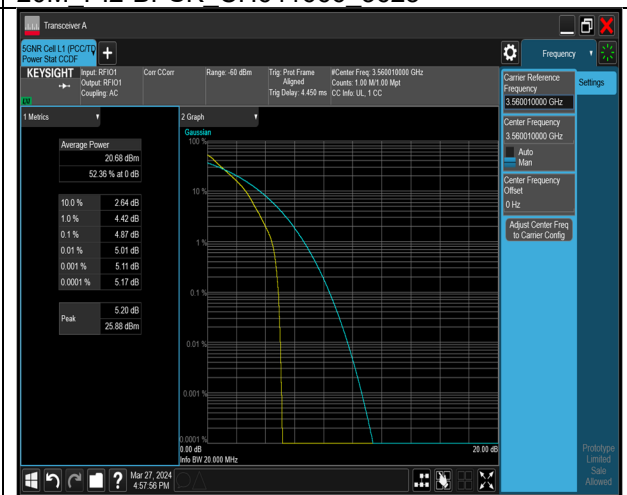
20M QPSK CH637334 3560
