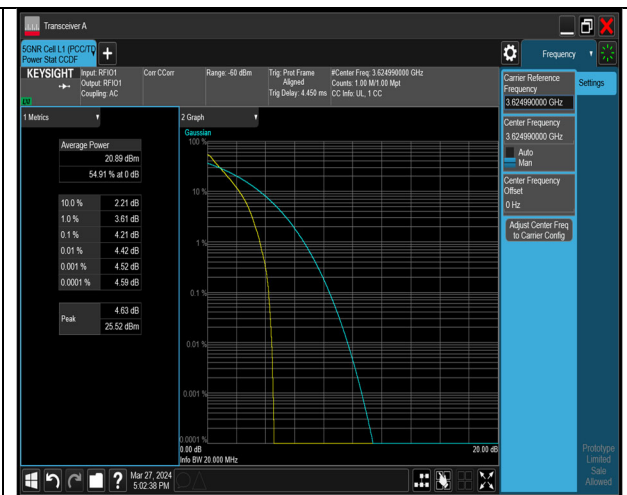
20M PI2-BPSK CH641666 3625
