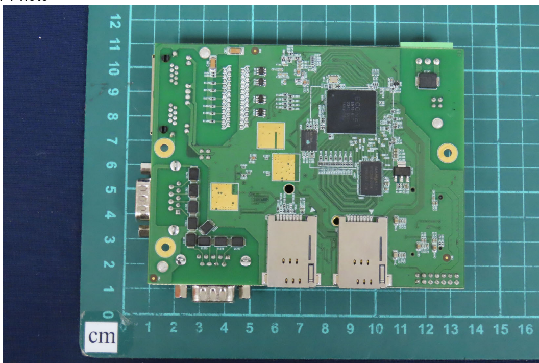
(15) EUT Photo
