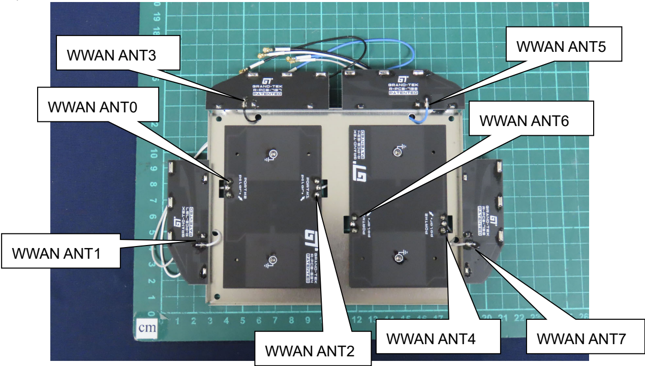
(24) EUT Photo
