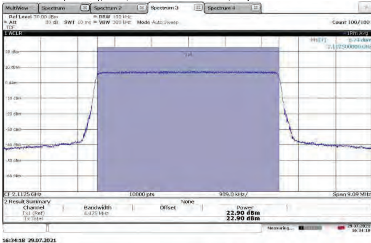
TM1.1-QPSK_5 MHz Bandwidth
