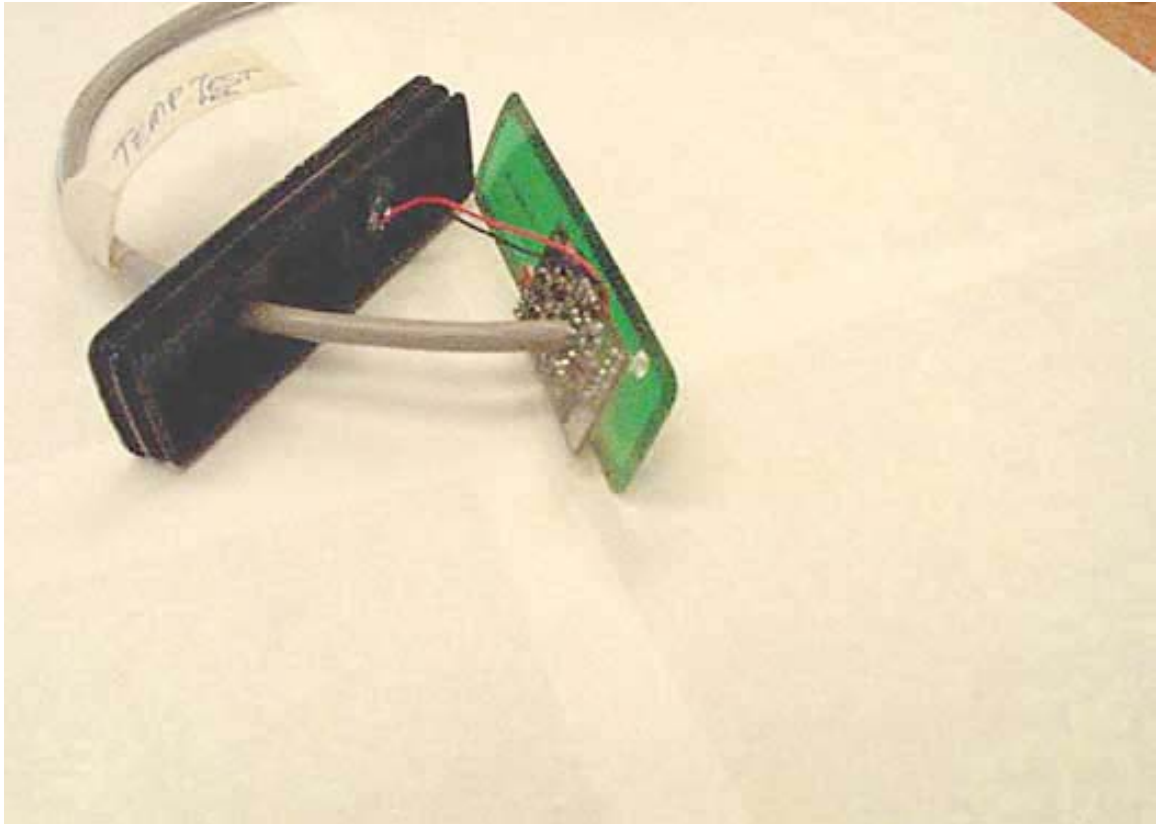
EUT Open
