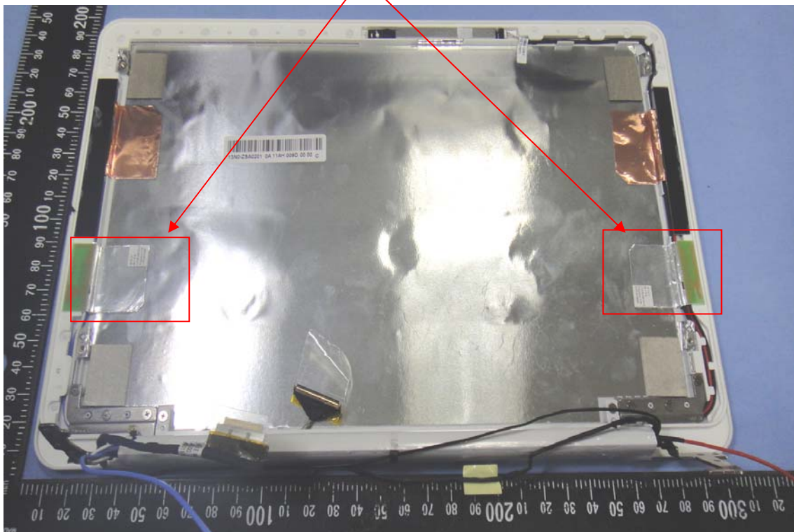
PIFA Antenna
