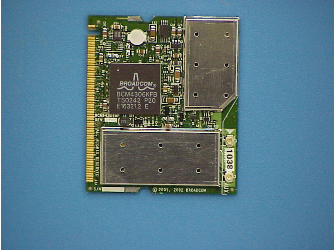
Photo 1. EUT top
