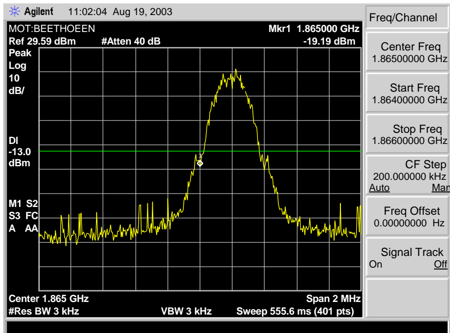
GSM 1900 D Min. Block Edge
