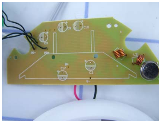
PCB1 side2
