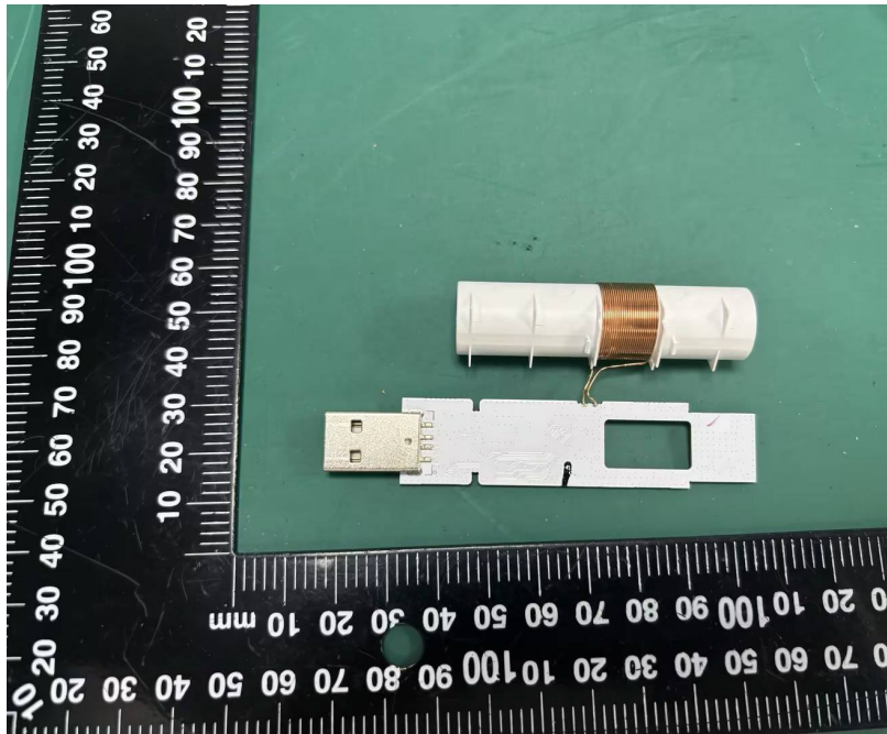
BLE Antenna
