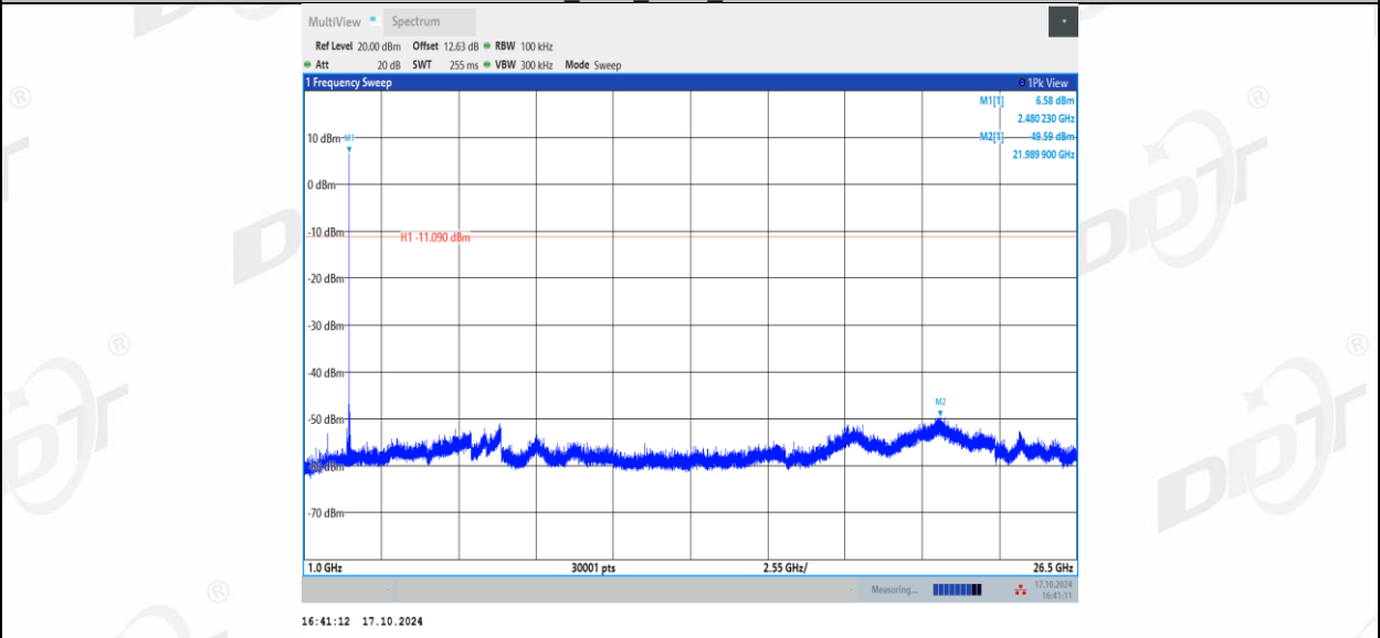
SRD Ant1 2480 1000~26500
