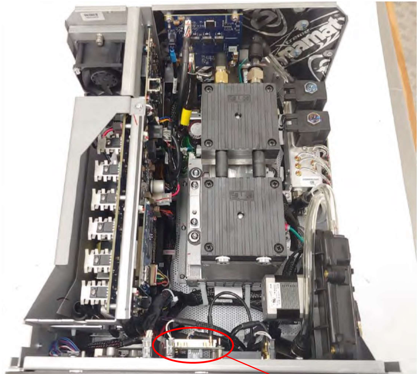
4 Channel RFID Module (5400-052-020)
