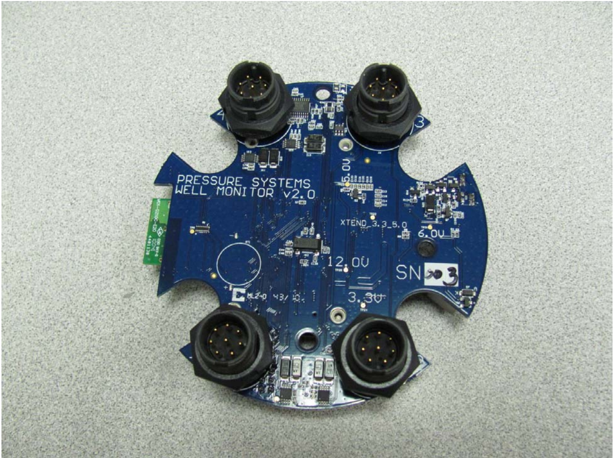
Node PCB Bottom
