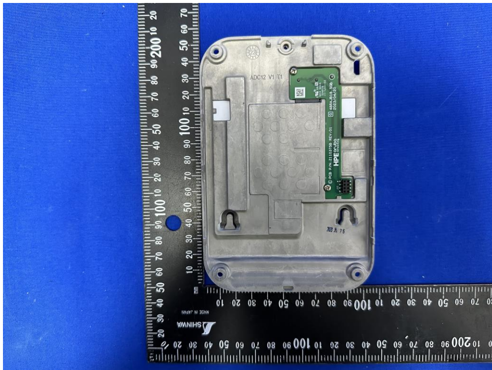
EUT Photo
