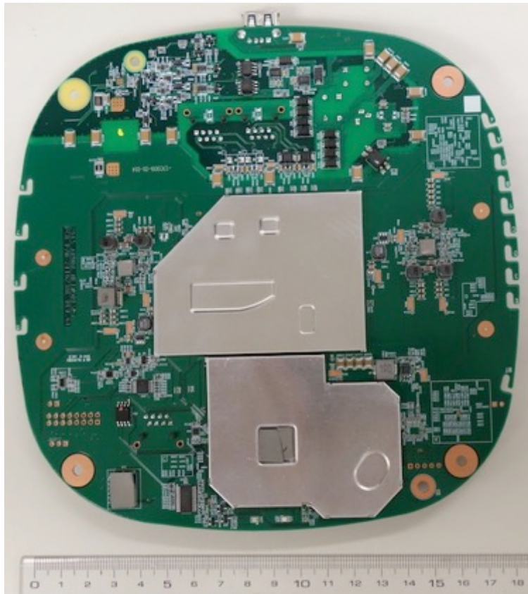
PCB - Bottom
