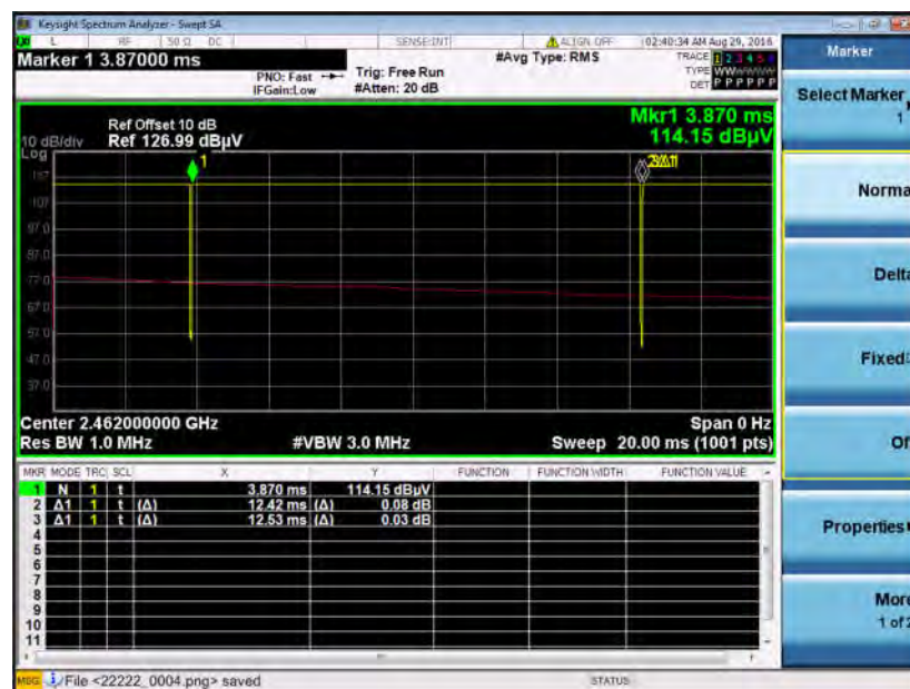
802.11b Antenna 1+2
