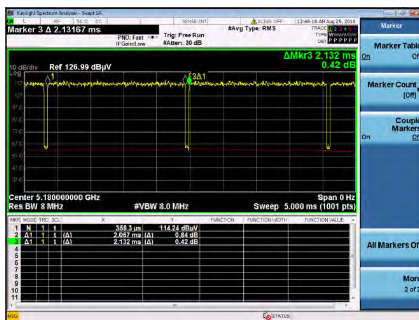
802.11a Antenna 1+2+3
