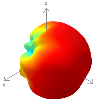
A3_BLE_6G 2.45GHz BLE antenna patterns
