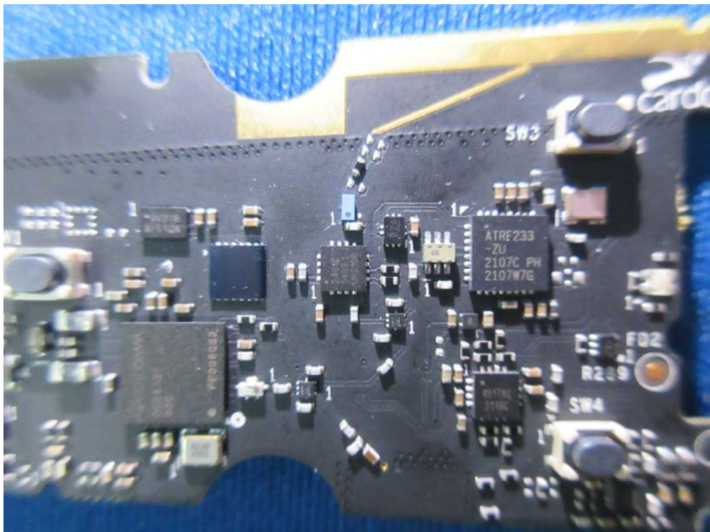
(12) EUT Photo
