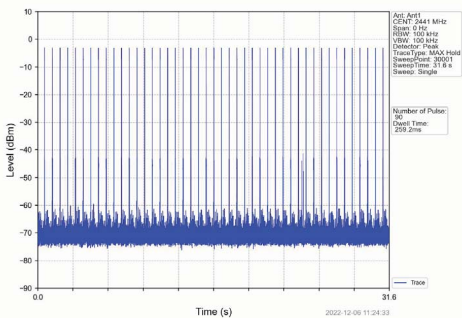
Pi/4DQPSK_2DH5_HOPP_Ant1_NTNV
