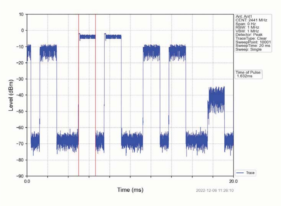
Pi/4DQPSK_2DH3_HOPP_Ant1_NTNV
