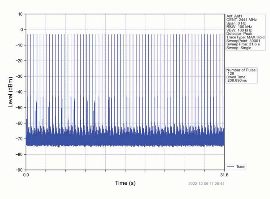
Pi/4DQPSK_2DH3_HOPP_Ant1_NTNV
