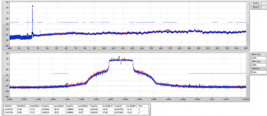
802.11g-BF_Nss1,(6Mbps)_2TX 2437MHz
