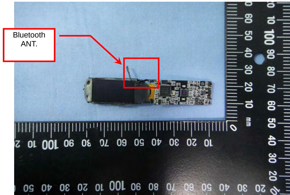
EUT Photo 11 )
