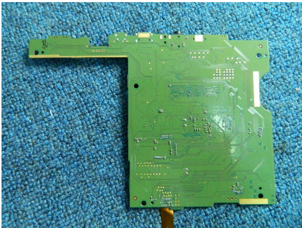
Mainboard (obverse)
