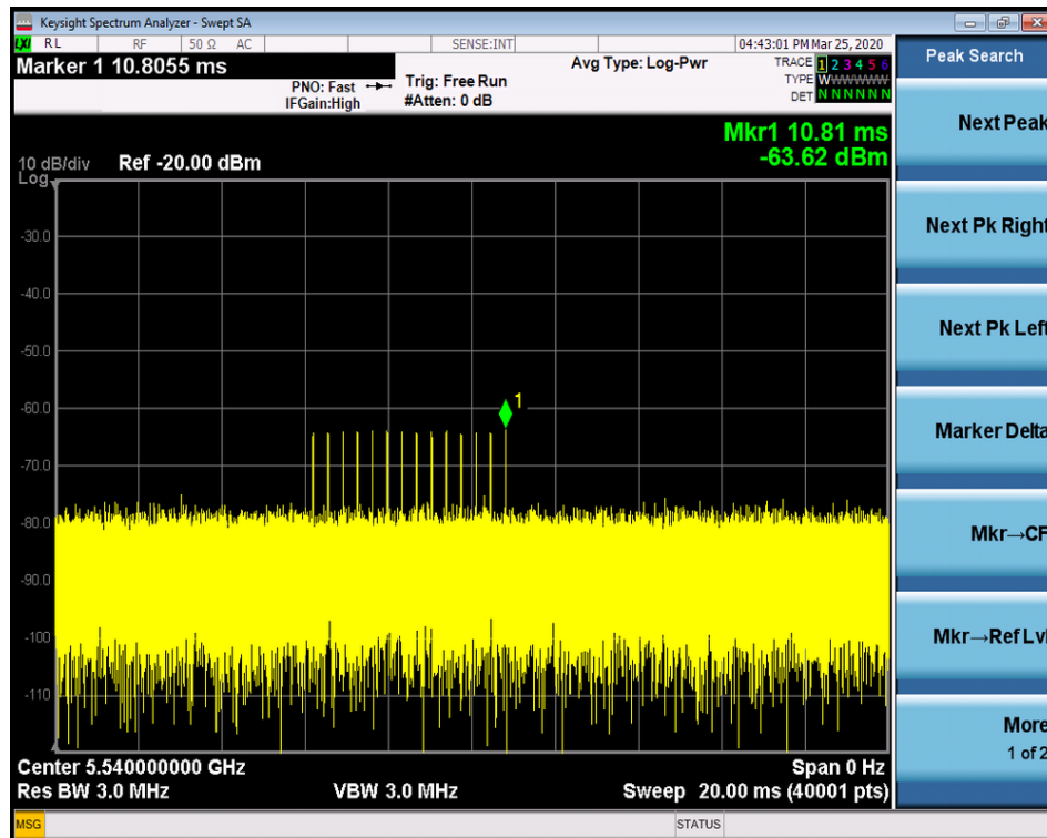
Radarsignal 5
