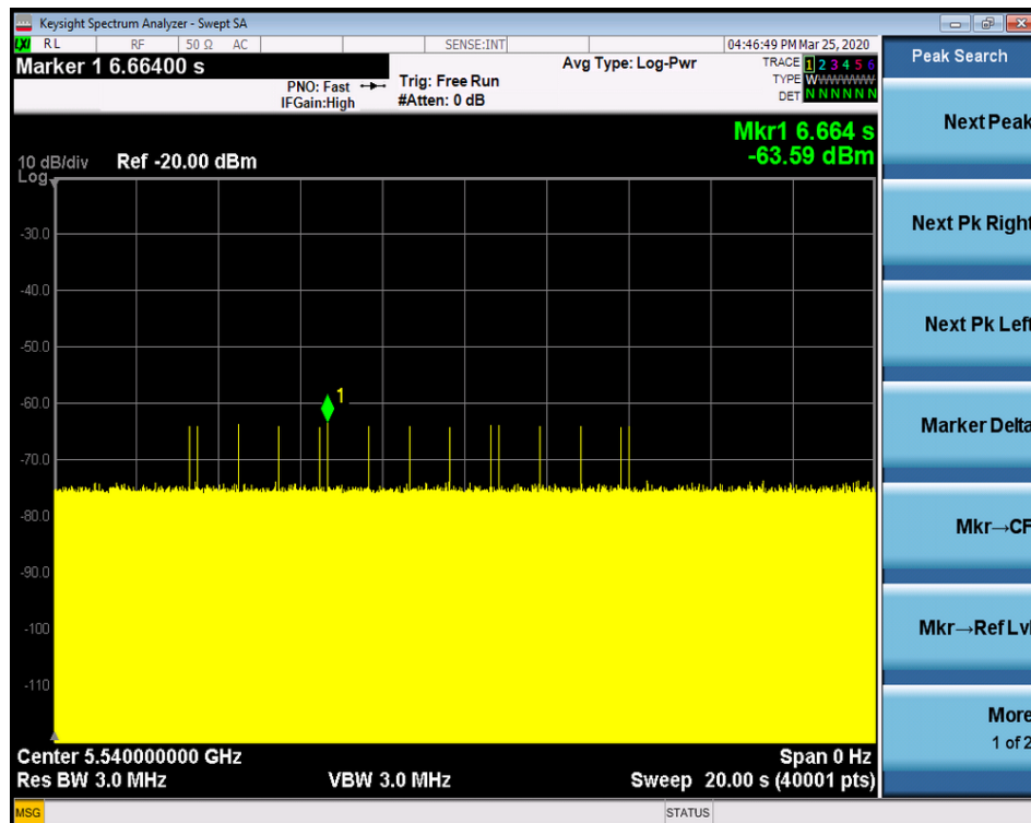
Radarsignal 5
