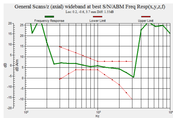
Fig. 8.8 CDMA2000 BC10 Ch580
