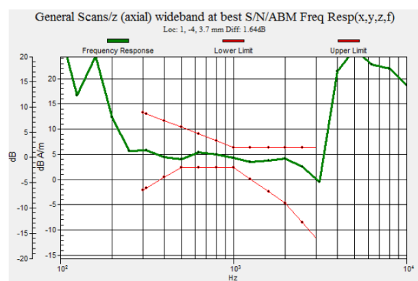
Fig. 8.6 CDMA2000 BC1 Ch1175
