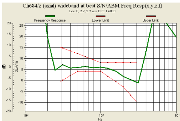
Fig. 8.9 CDMA2000 BC10 Ch684
