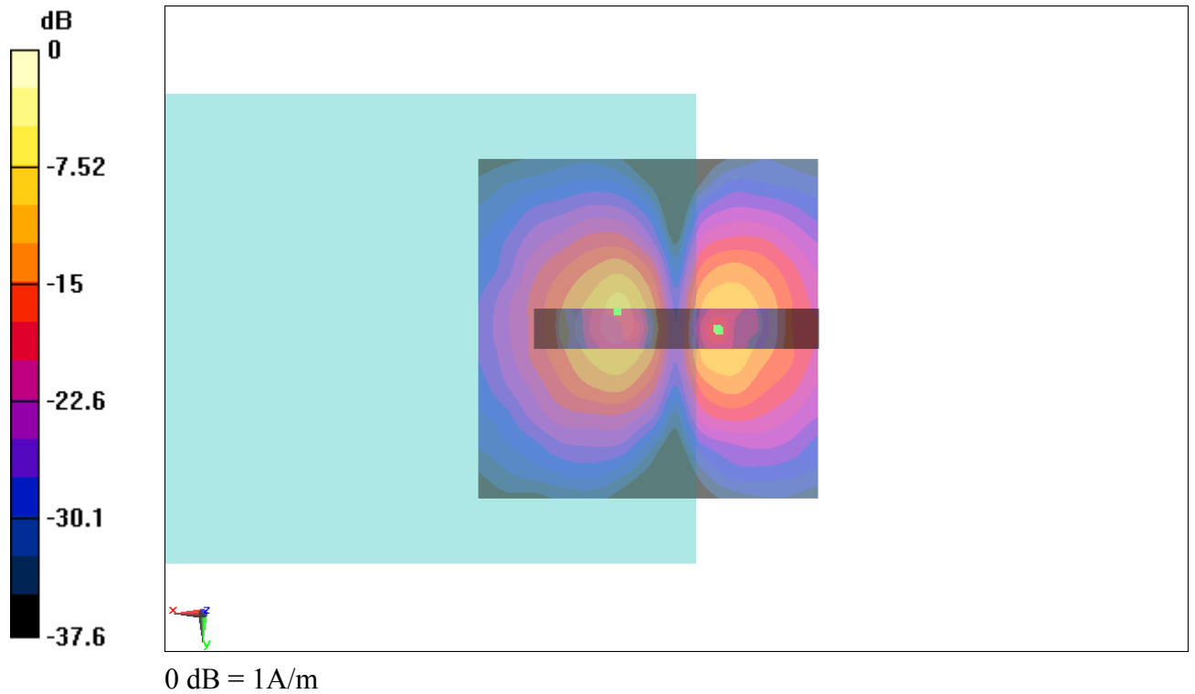
Fig B.4 T-Coil CDMA 835_Channel 384
