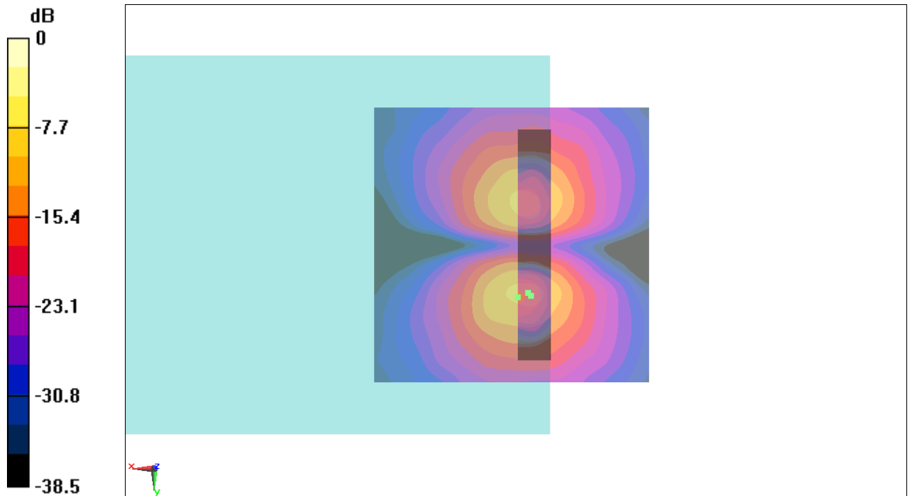
Fig B.5 T-Coil CDMA 835_Channel 384
