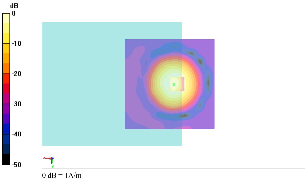
Fig B.6 T-Coil CDMA 835_Channel 384
