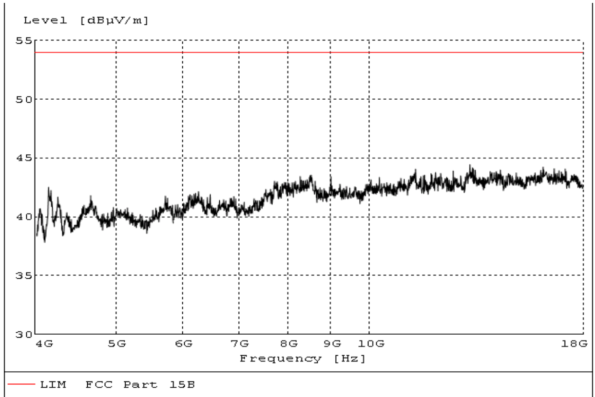
(WCDMA Band V: 4GHz-18GHz)
