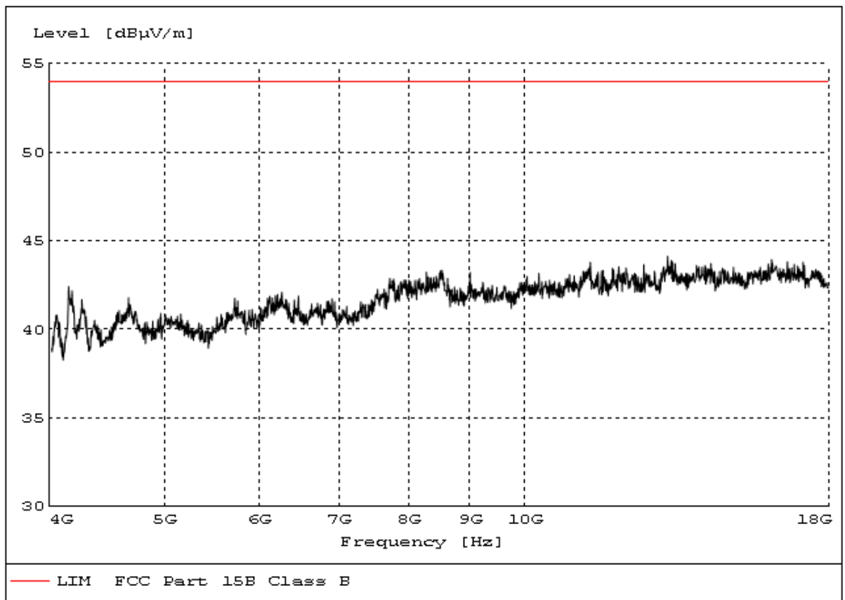
(WCDMA Band II: 4GHz-18GHz)
