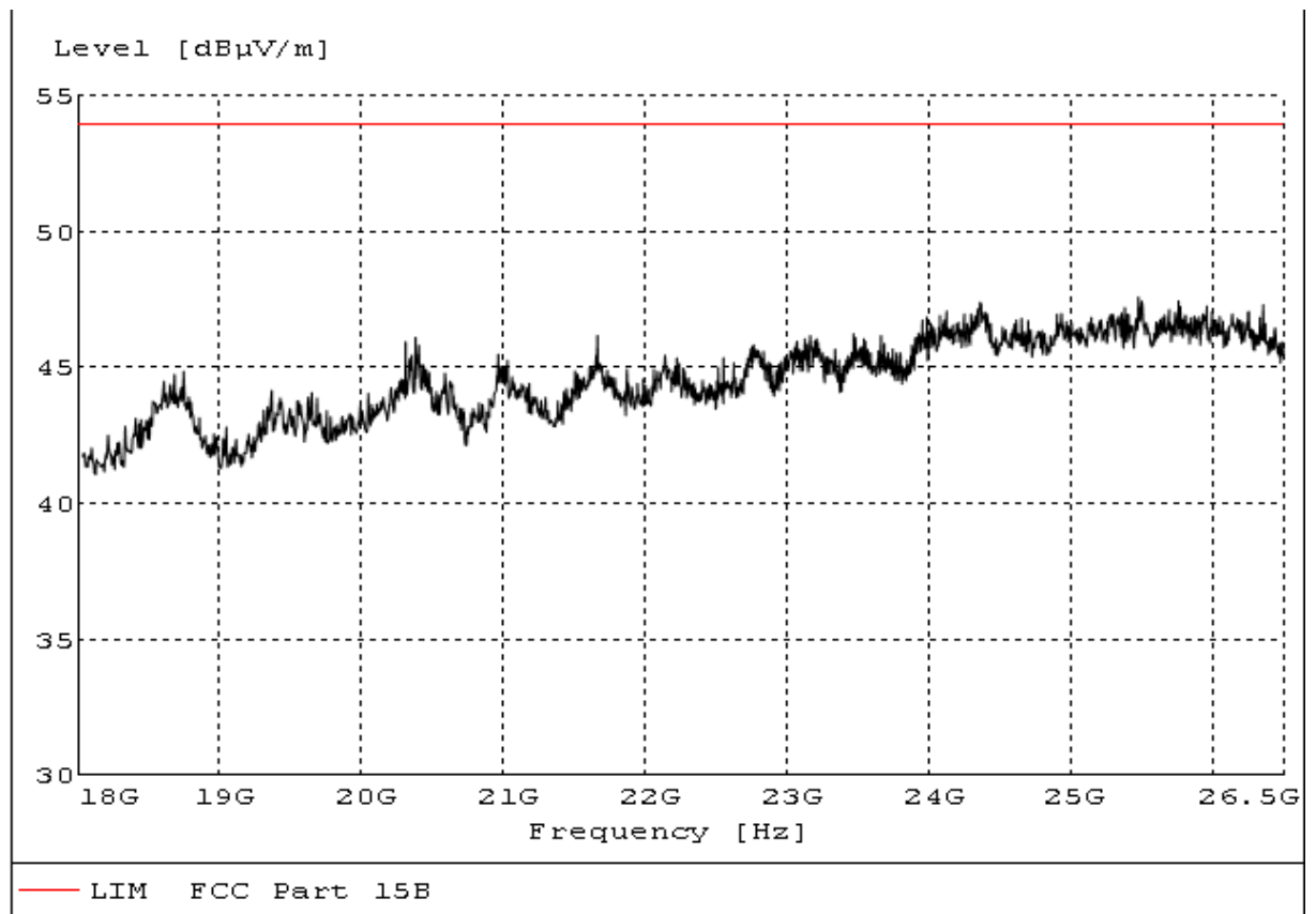
(WCDMA Band V: 18GHz-26.5GHz)
