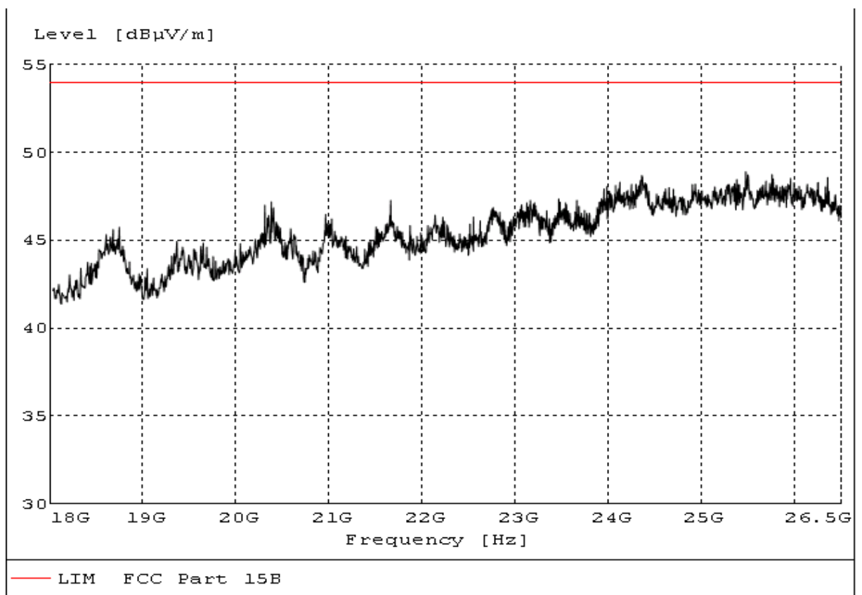
(WCDMA Band II: 18GHz-26.5GHz)
