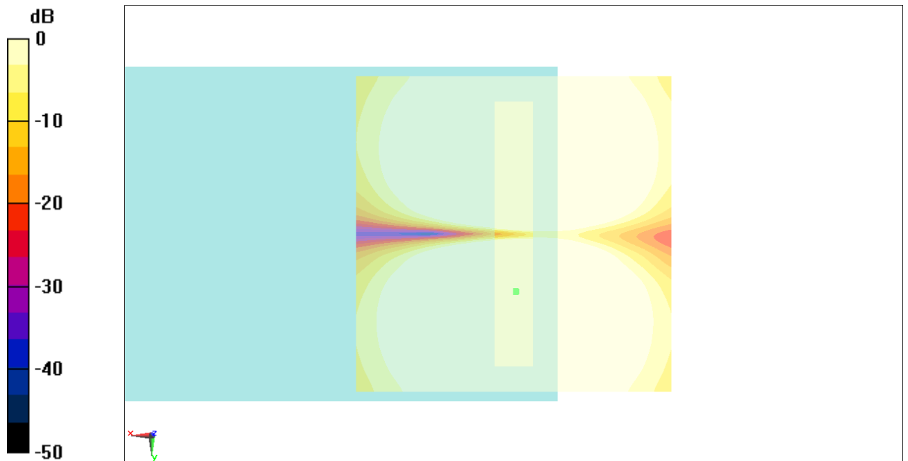
Fig B.11 T-Coil WCDMA 1900
