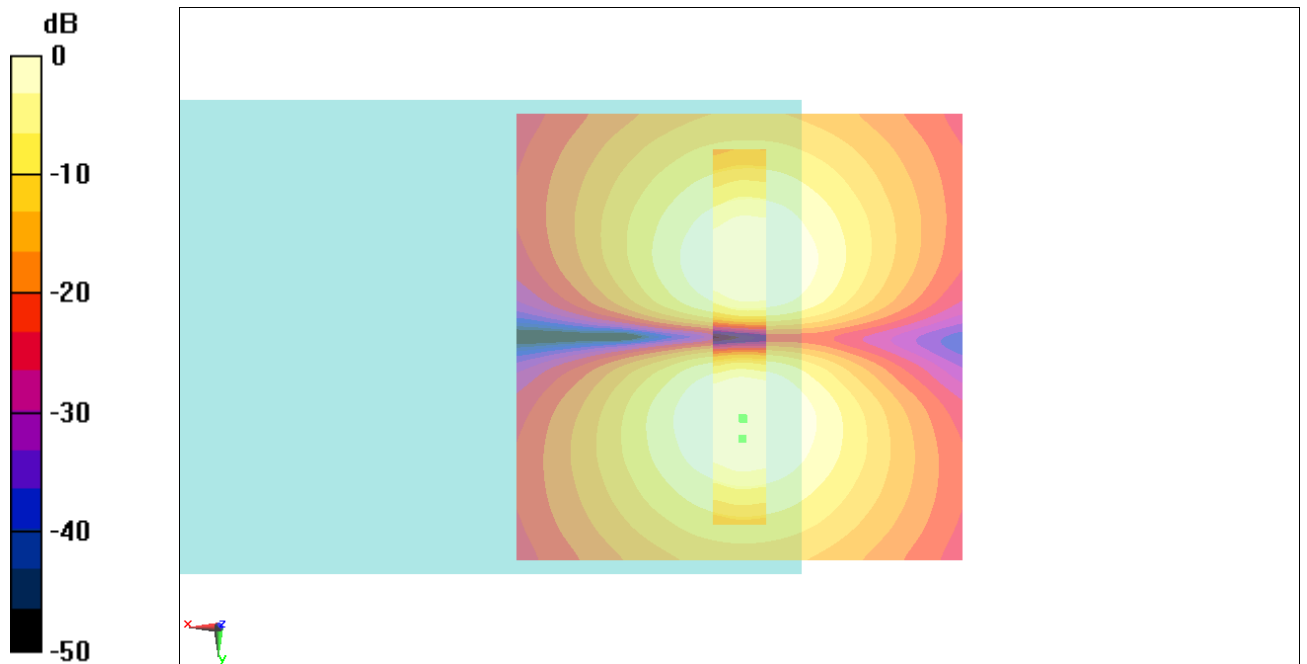
Fig B.8 T-Coil WCDMA 850
