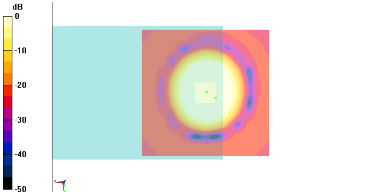
Fig B.9 T-Coil WCDMA 850
