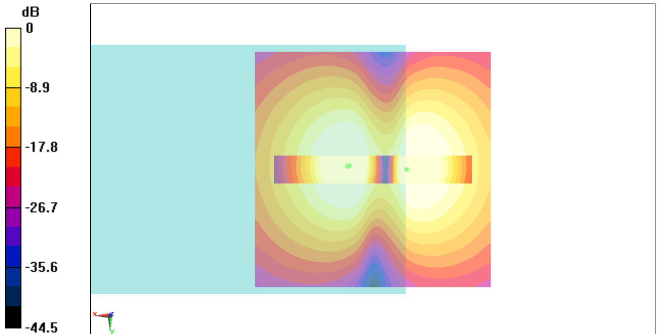
Fig B.7 T-Coil WCDMA 850
