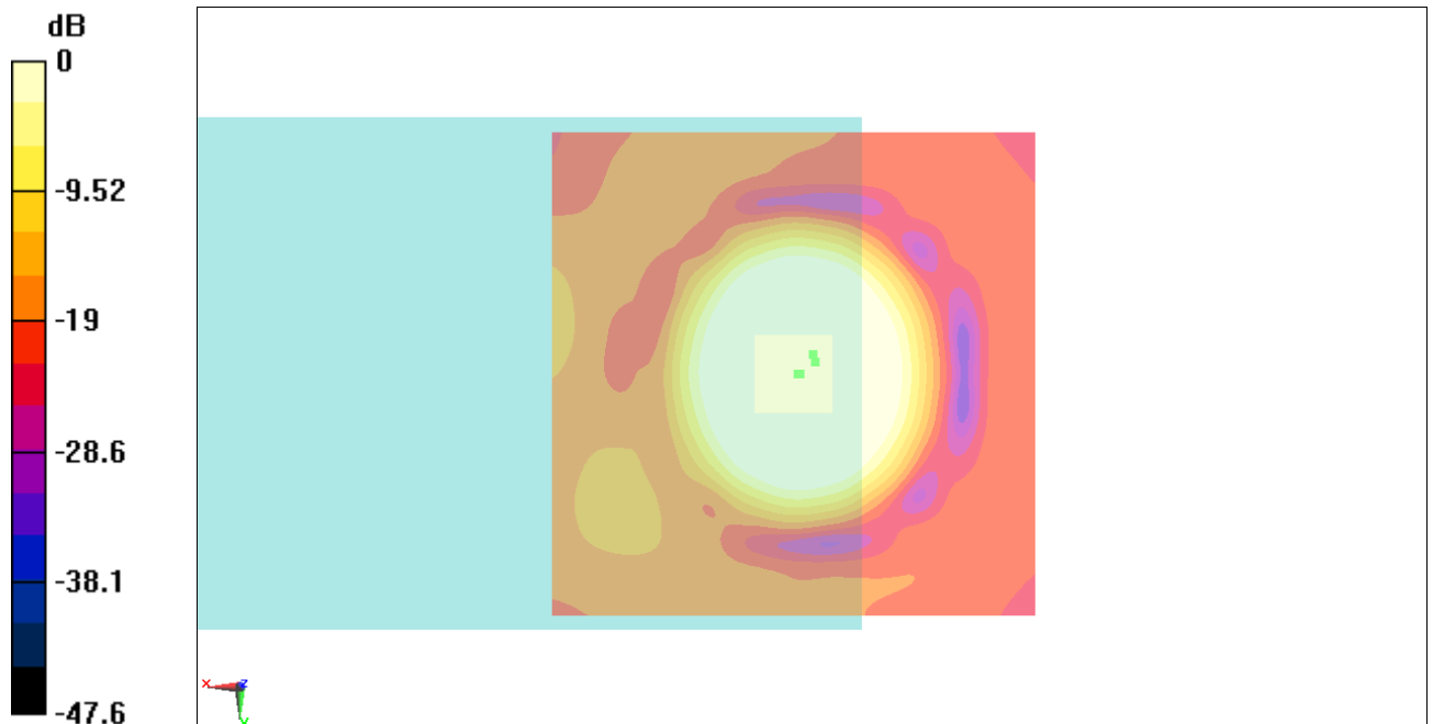
Fig B.3 T-Coil GSM 850
