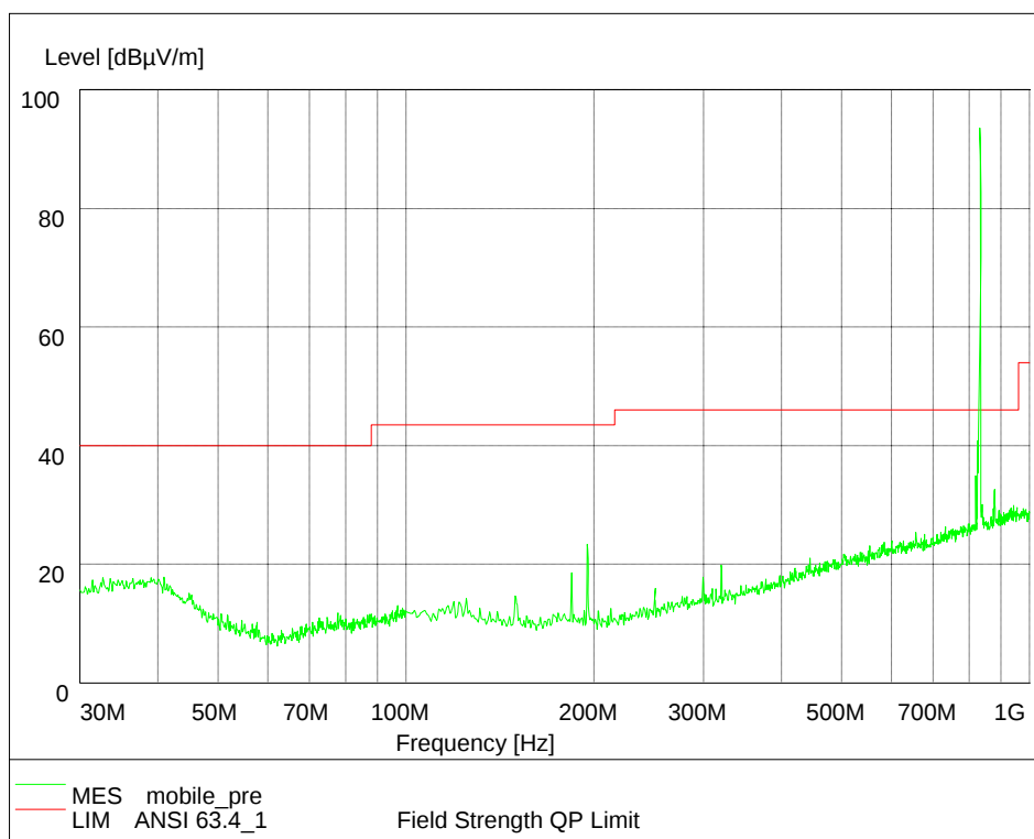
Pic.3 CDMA 1X (30MHz – 1GHz)
