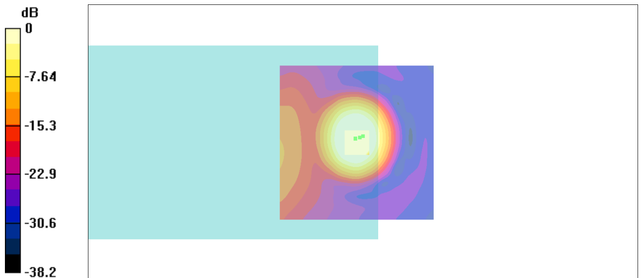
Fig B.3 T-Coil GSM 850
