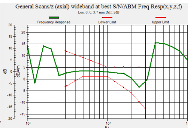
Fig 8.2 GSM850 Ch189
