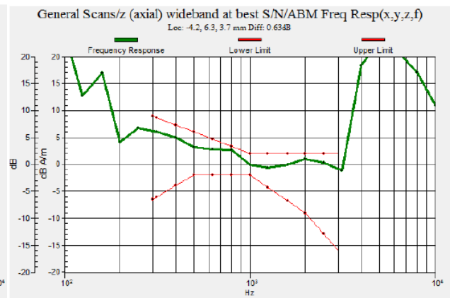
Fig 8.2 GSM850 Ch189
