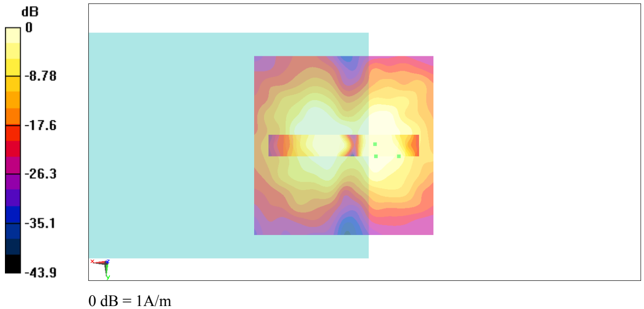
Fig B.7 T-Coil WCDMA 850
