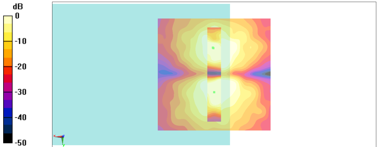
Fig B.8 T-Coil WCDMA 850
