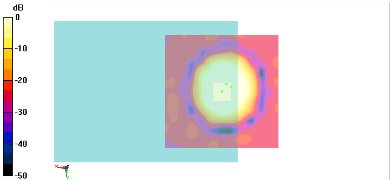
Fig B.9 T-Coil WCDMA 850
