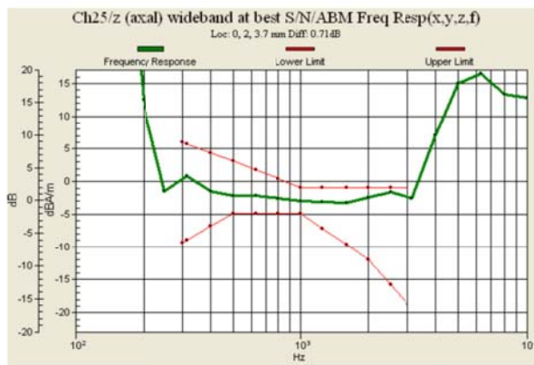
Fig 8.4 CDMA2000 BC1 Ch25
