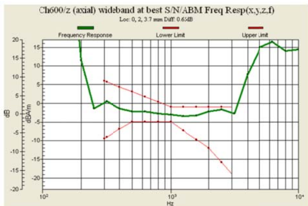
Fig 8.5 CDMA2000 BC1 Ch600
