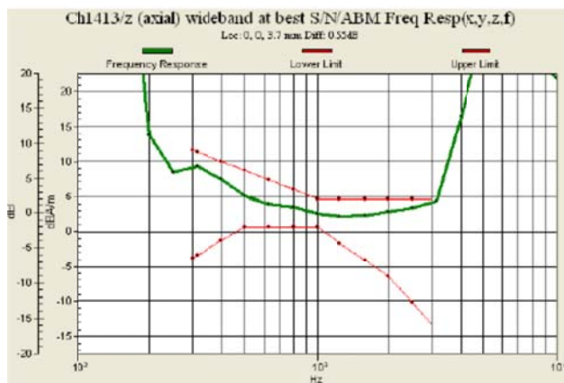
Fig. 8.11 WCDMA Band IV Ch1413
