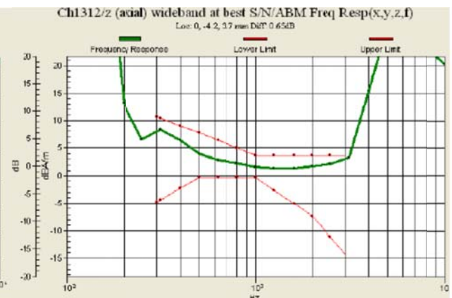
Fig. 8.10 WCDMA Band IV Ch1312
