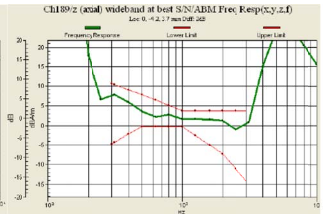
Fig 8.2 GSM850 Ch189
