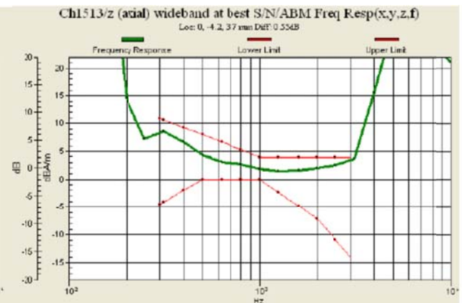
Fig. 8.12 WCDMA Band IV Ch1513
