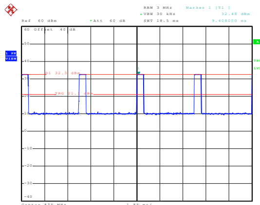
835MHz - GSM
