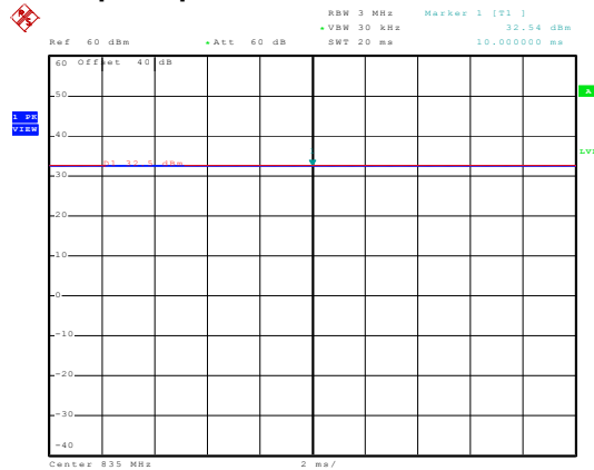
835MHz - CW
