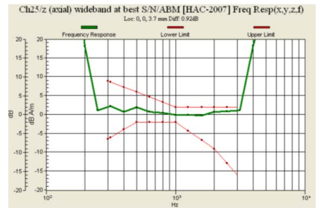
Fig. 9.4 CDMA2000 BC1 Ch25
