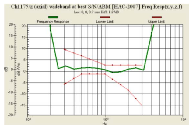
Fig. 9.6 CDMA2000 BC1 Ch1175
