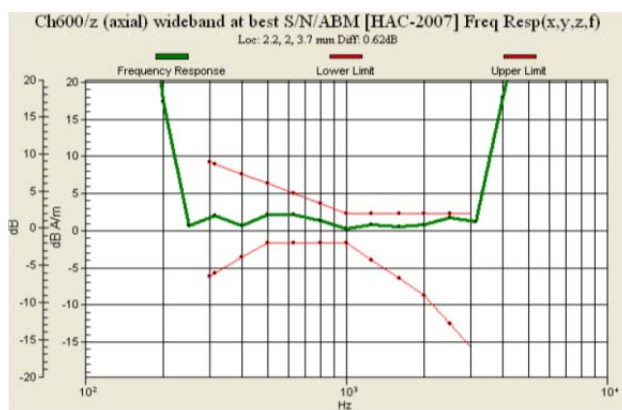
Fig. 9.5 CDMA2000 BC1 Ch600
