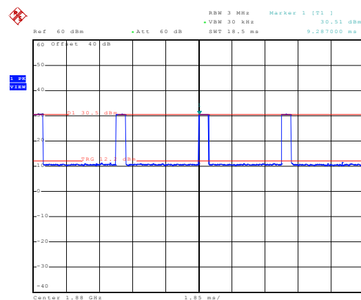
1880MHz - GSM
