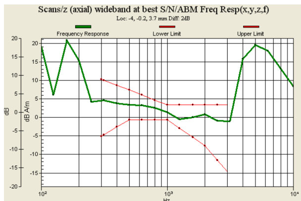
Fig. 9.9 CDMA2000 BC15 Ch875
